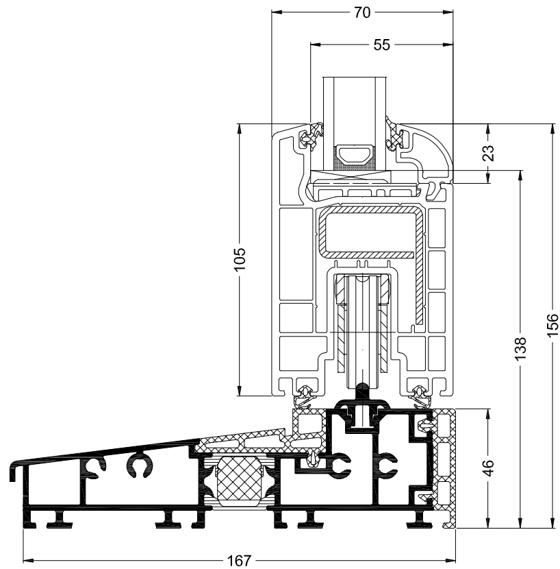
Schüco EasySlide
